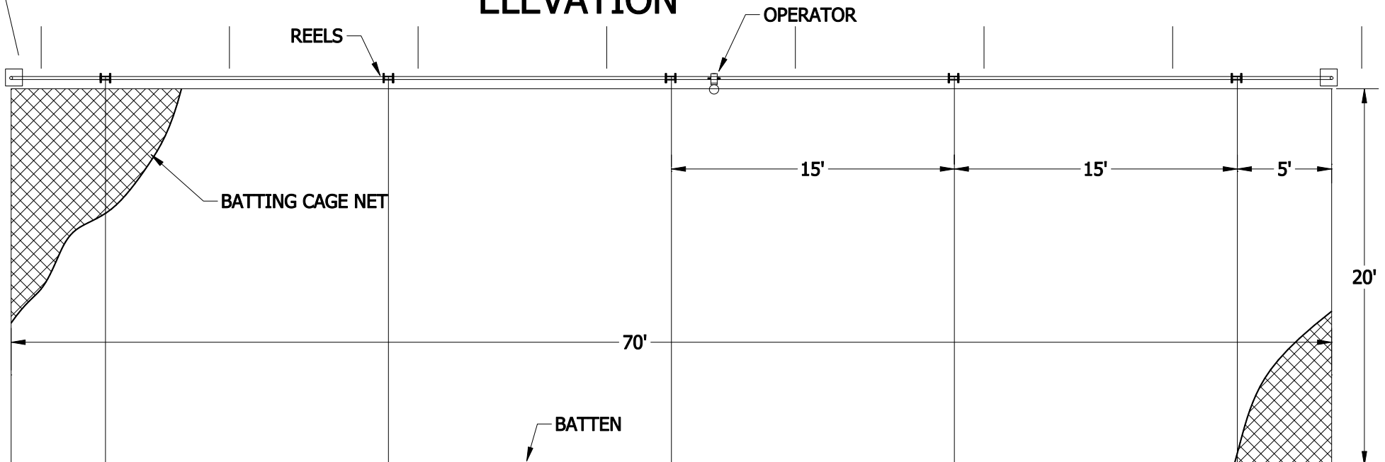
ELEVATION
