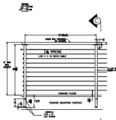
ELEVATION B
