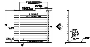
ELEVATION B
