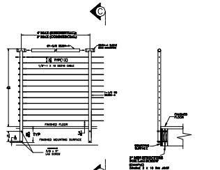
ELEVATION B
