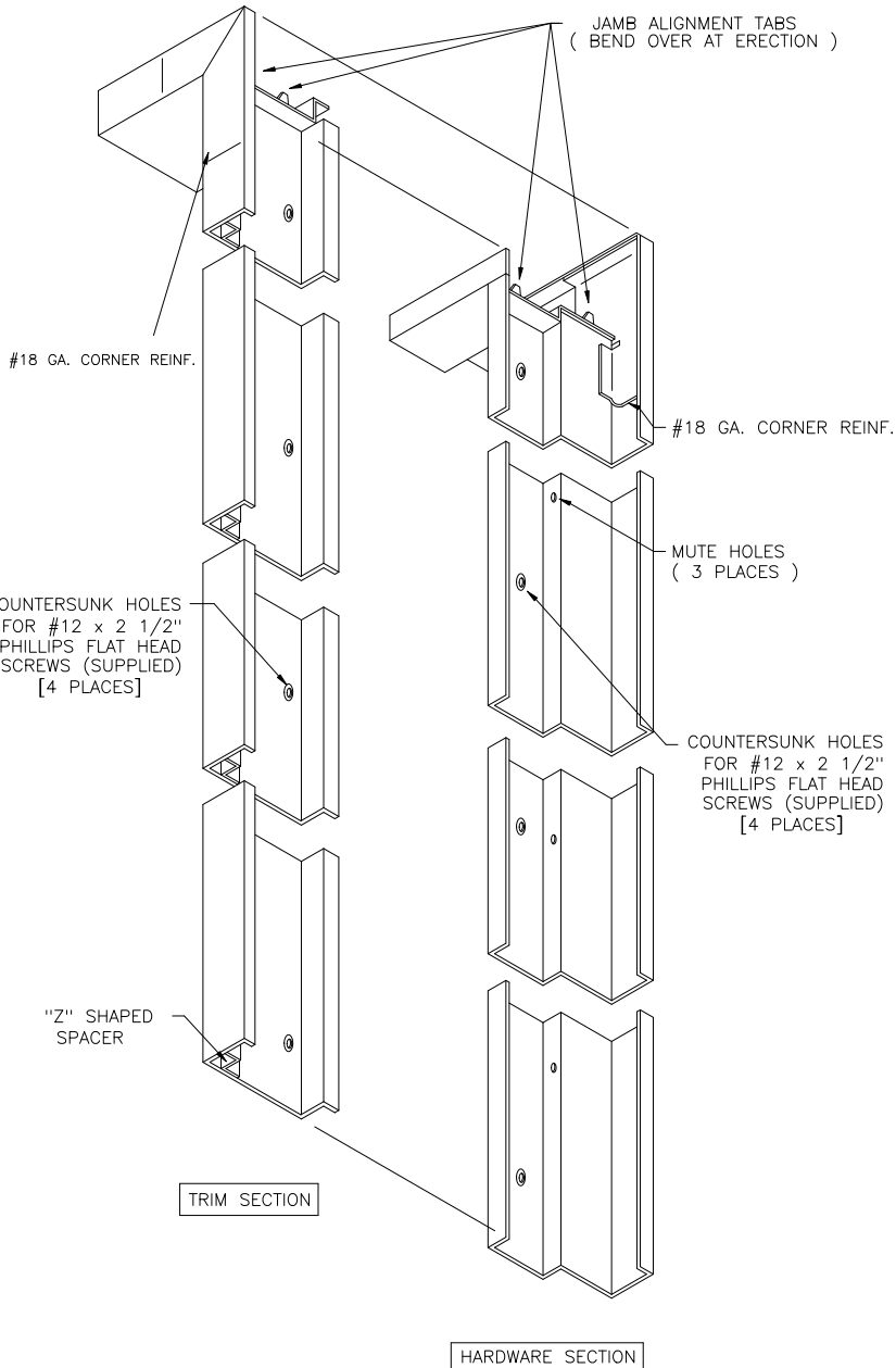
HDWRE SECTION
