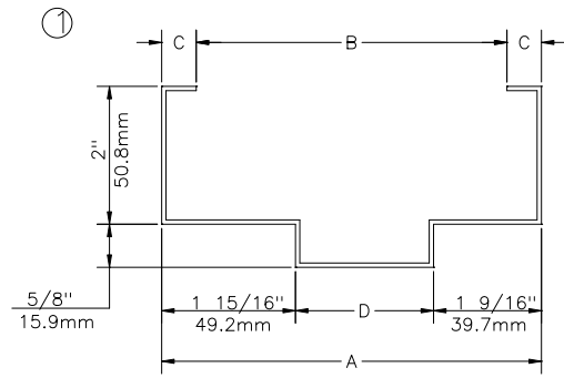
UNEQUAL RABBET
