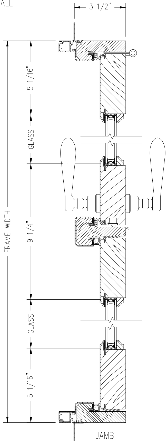
HORIZONTAL SECTION POST DOOR
