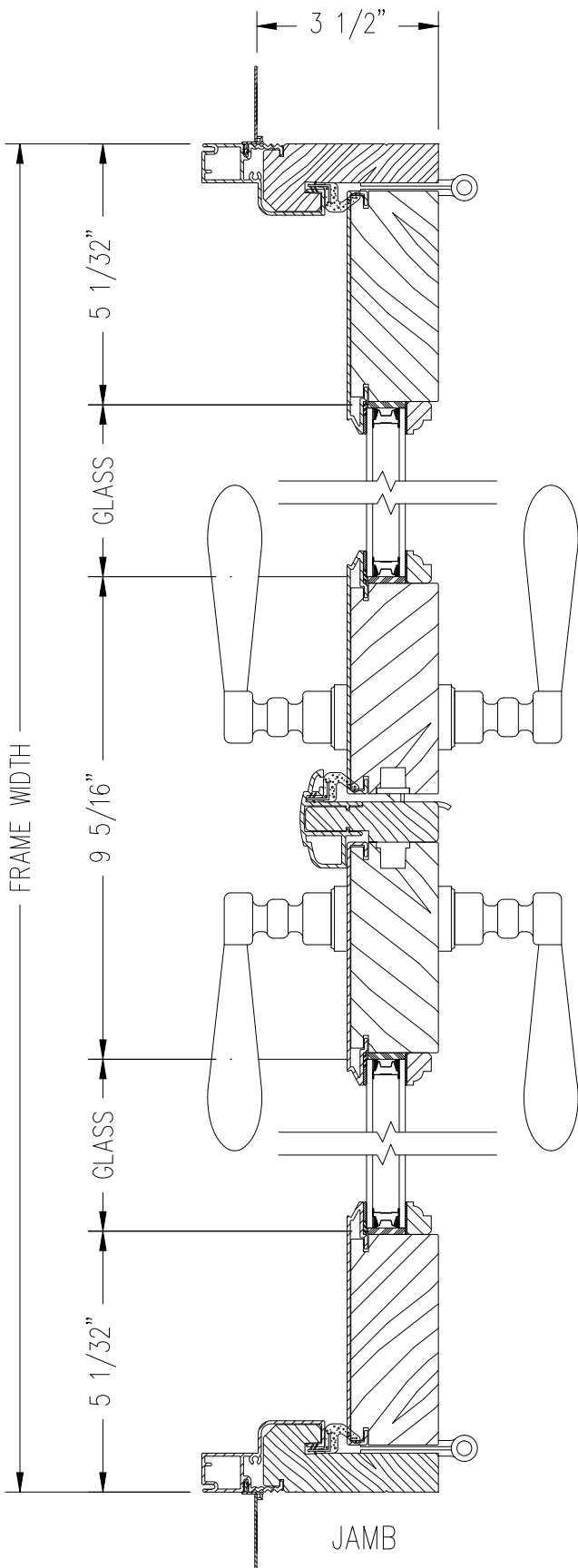
HORIZONTAL SECTION DOUBLE DOOR
