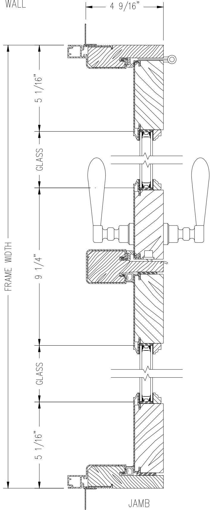
HORIZONTAL SECTION POST DOOR
