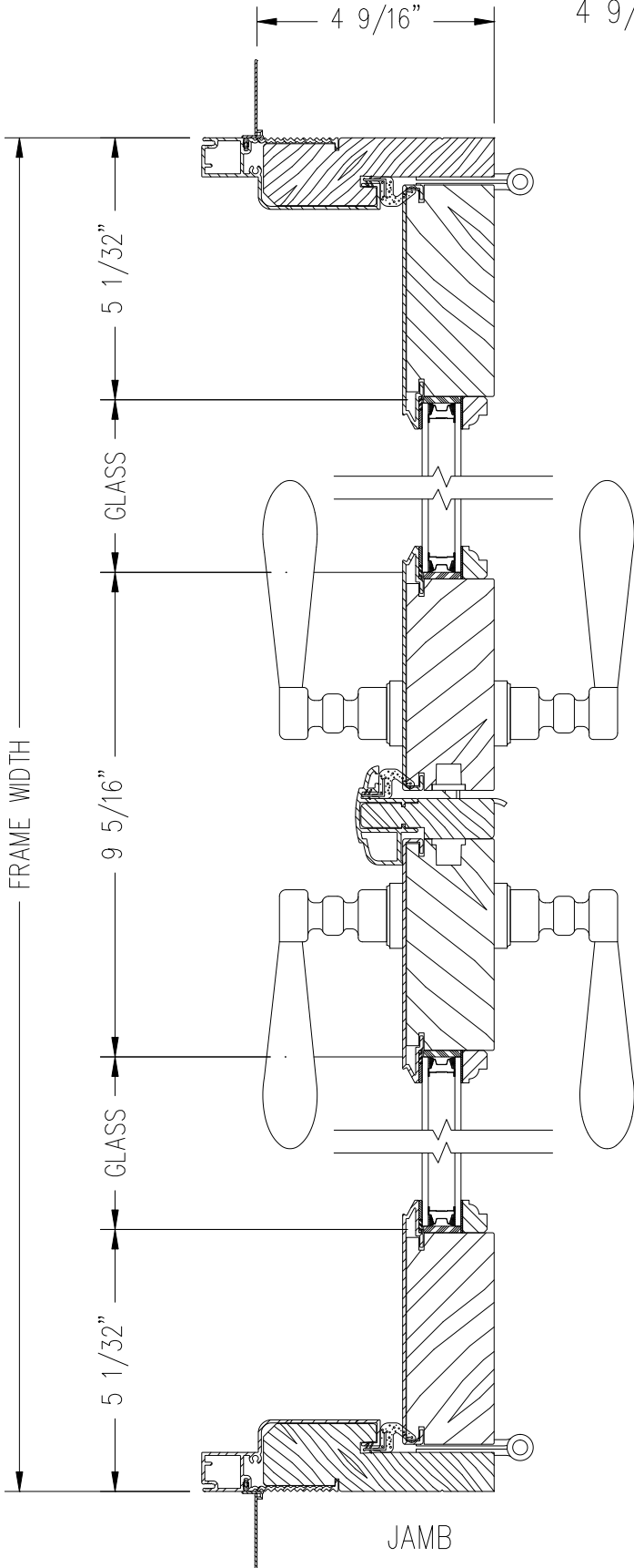
HORIZONTAL SECTION DOUBLE DOOR
