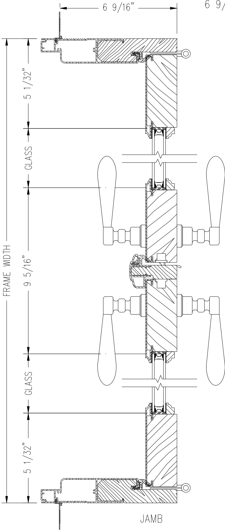
HORIZONTAL SECTION DOUBLE DOOR
