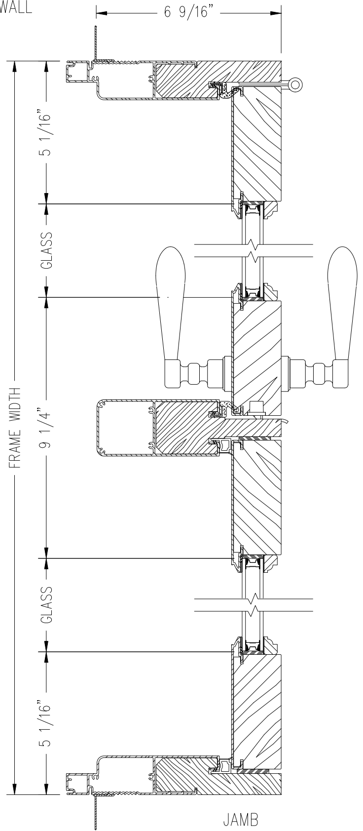
HORIZONTAL SECTION POST DOOR
