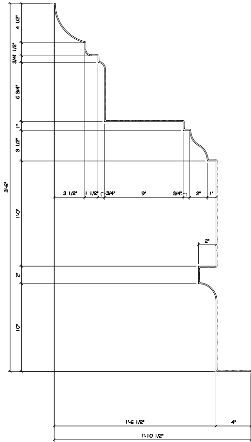
A SECTION THRU CR-150 4 SCALE: 3" = 1'-0"
