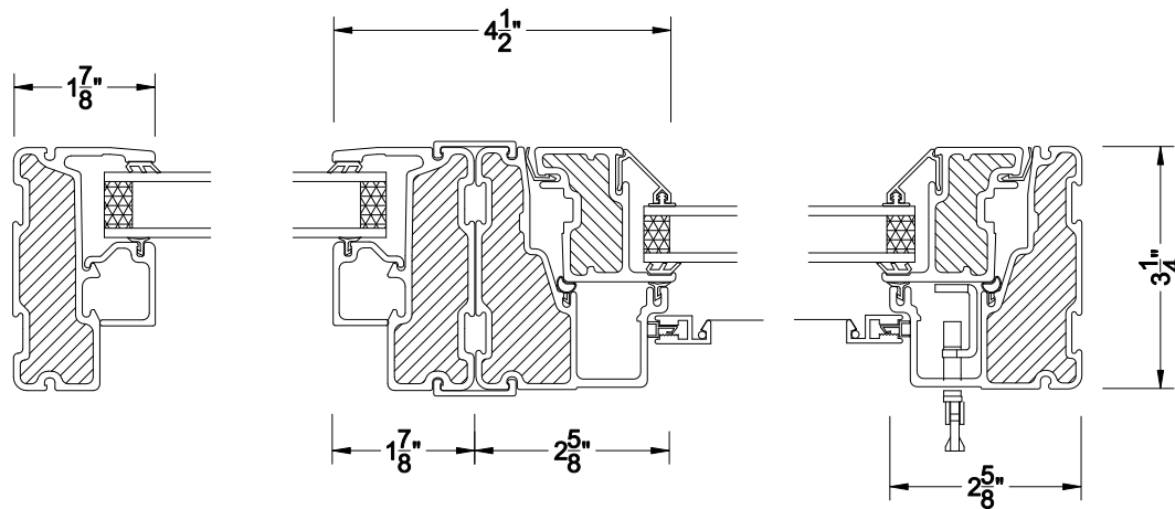
JAMB DETAIL
