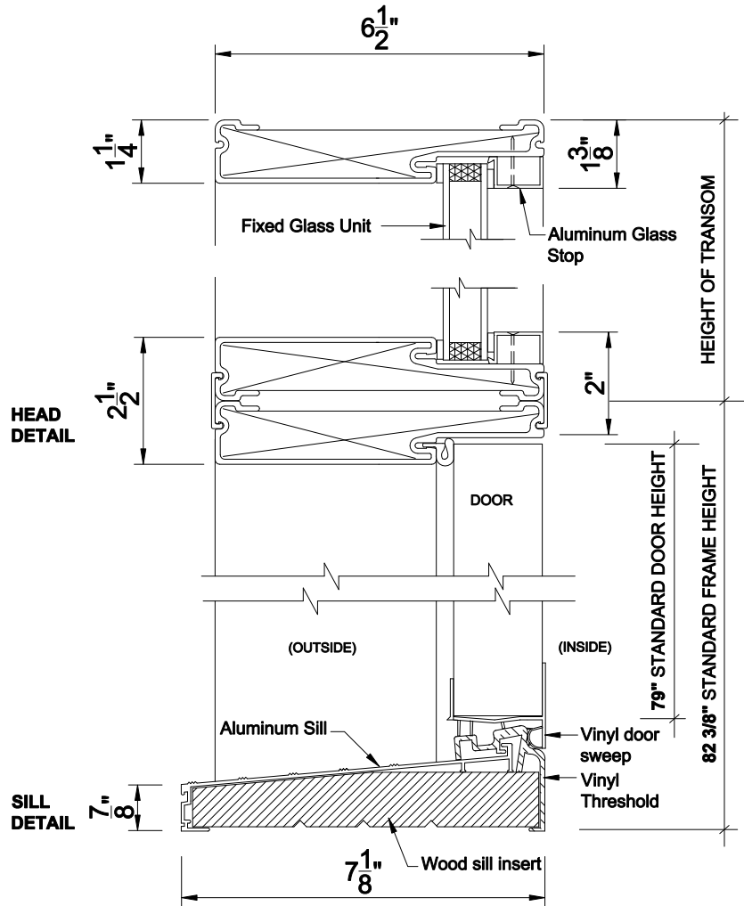
SECTION A-A
