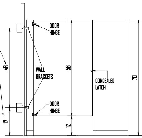
ELEV.: A
