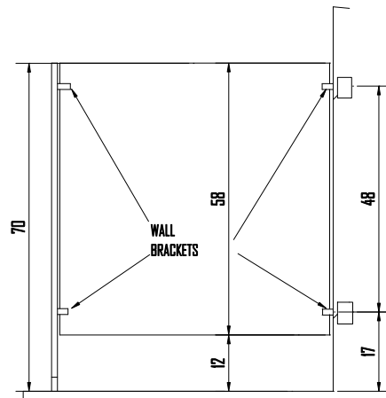
ELEV.: B
