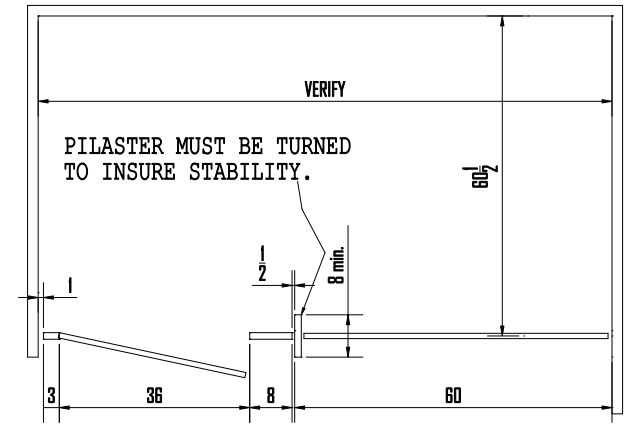
ADA-ALCOVE
