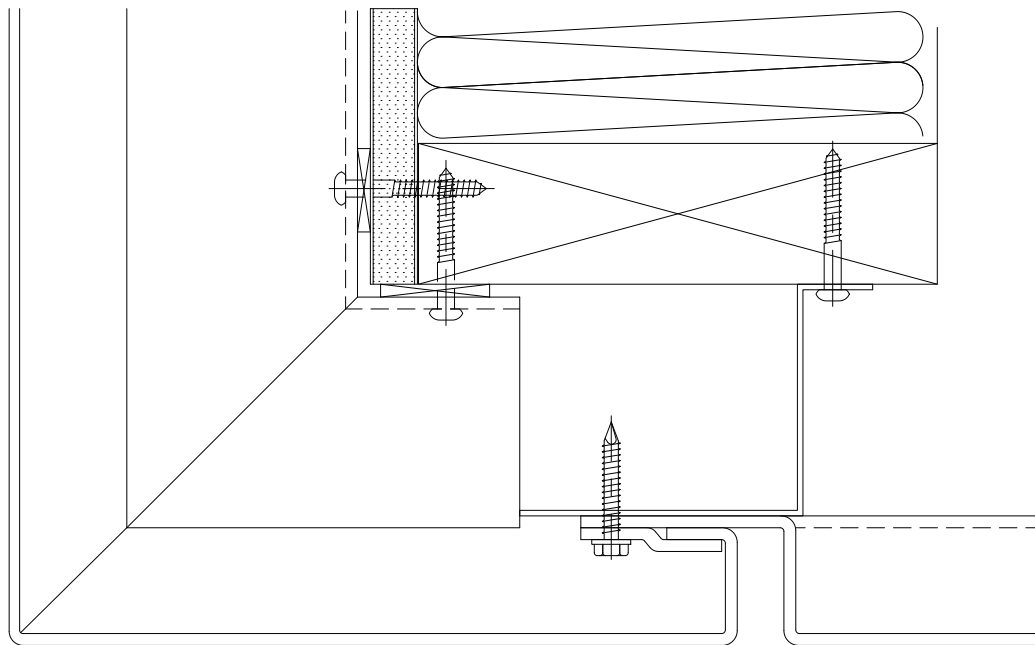
10. SOFFIT
