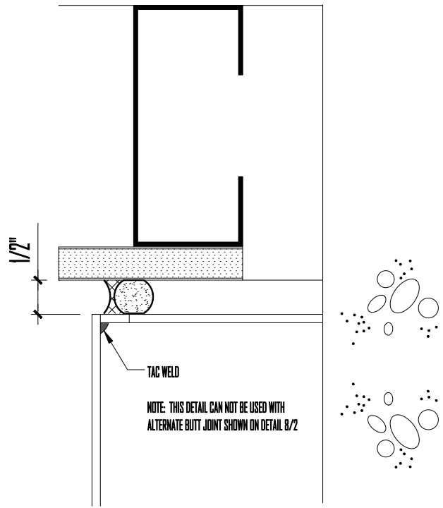
9A. TOP OF COVER
