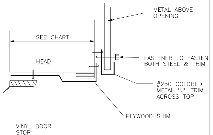
OVHEAD DOOR FLASHING
