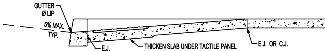
SECTION A-A
