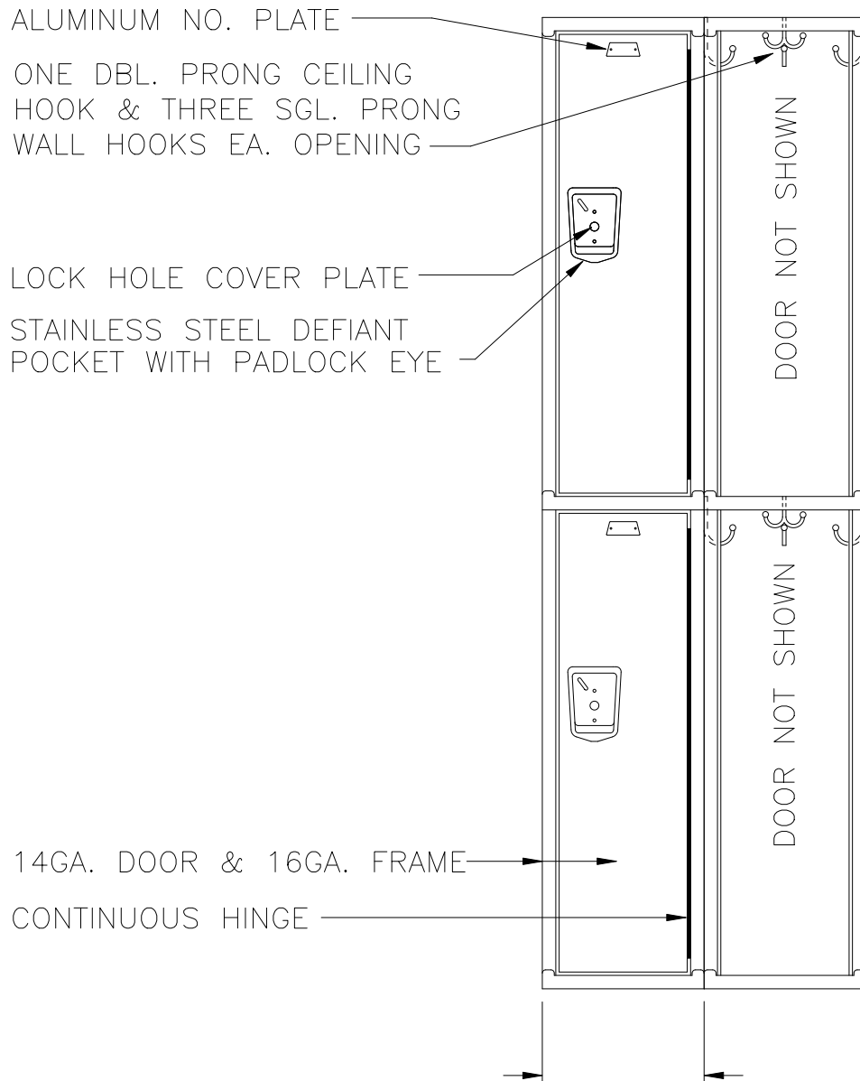
ELEVATION
