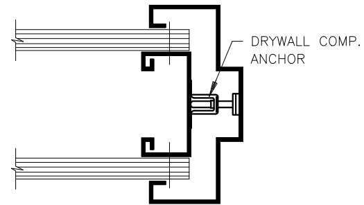
STEEL STUD WALL
