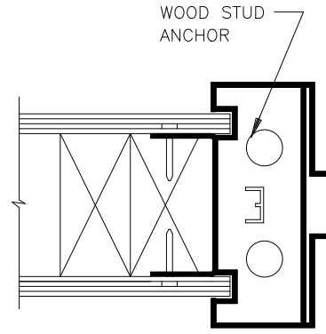
WOOD STUD WALL
