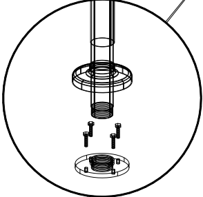
EXPLODED VIEW SCALE: N.T.S.
