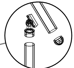
EXPLODED VIEW SCALE: N.T.S.
