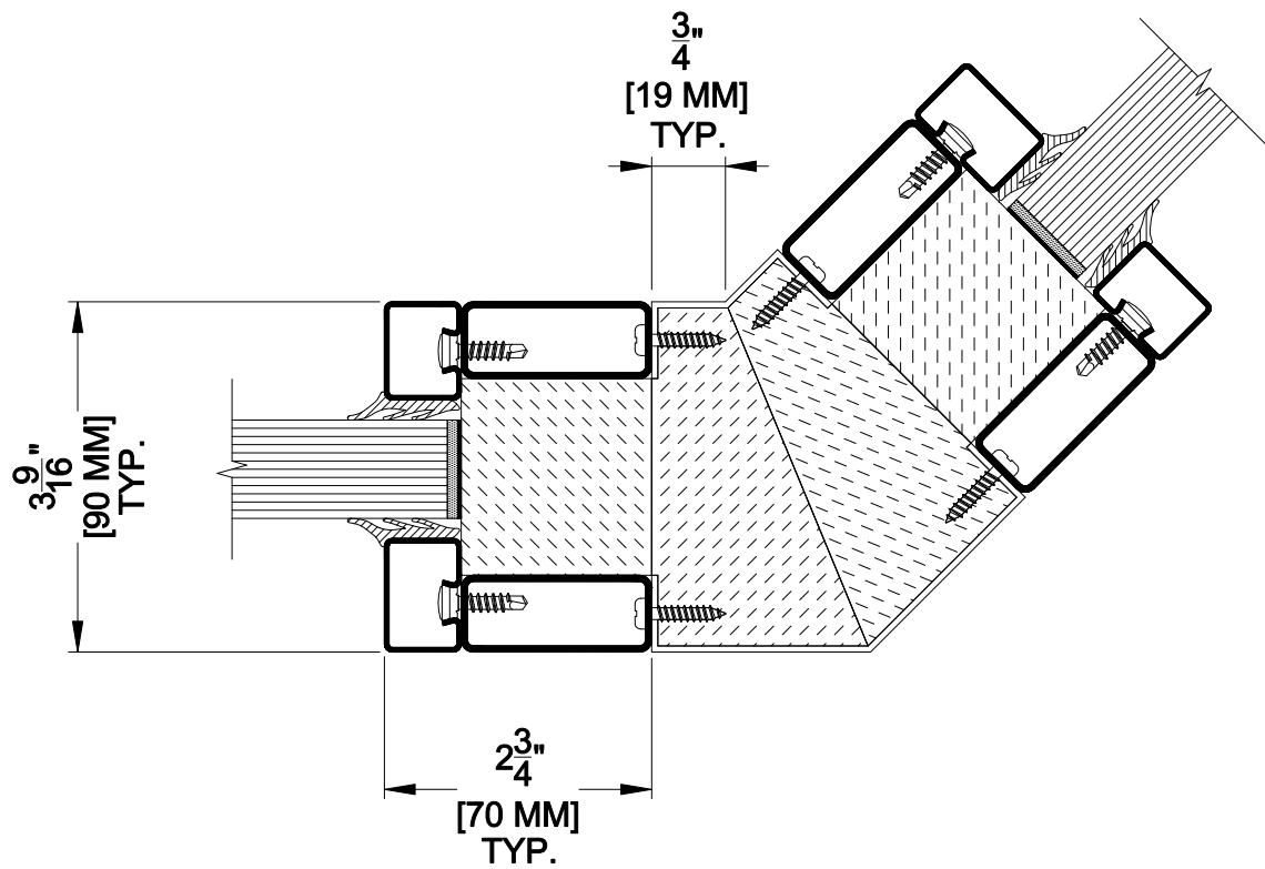
VDS-60 MIN. 45° OFFSET
