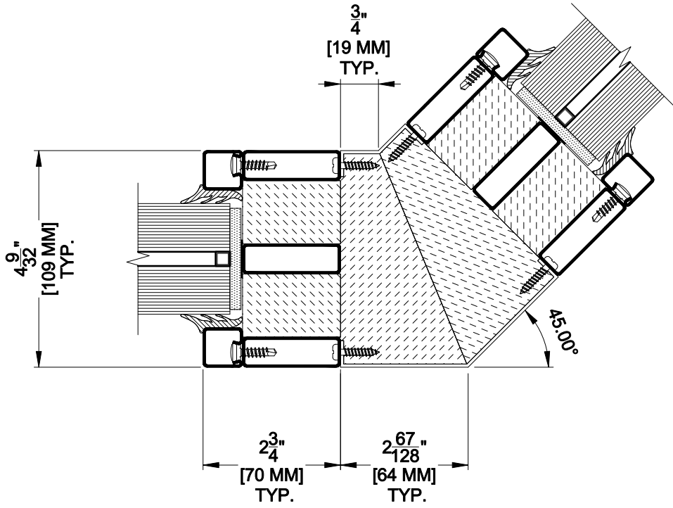
VDS-120 45° OFFSET
