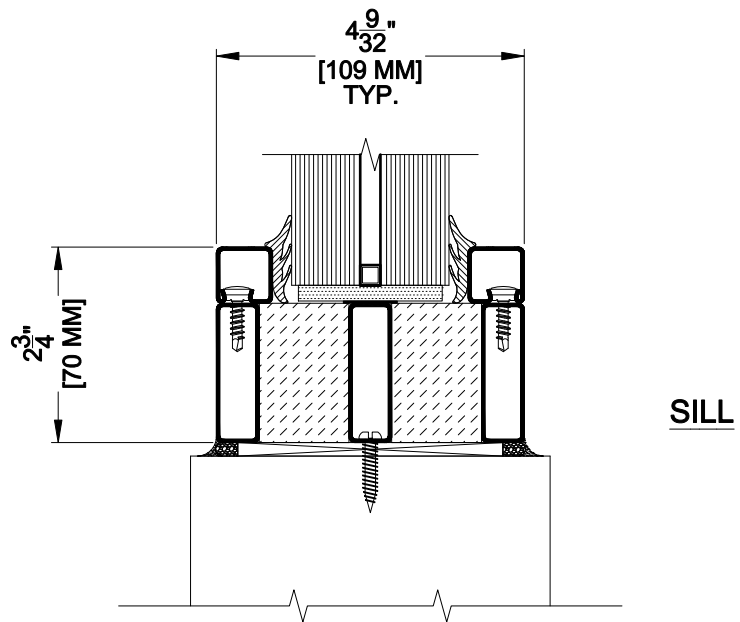
VDS-120 MIN. SECTION "CC"
