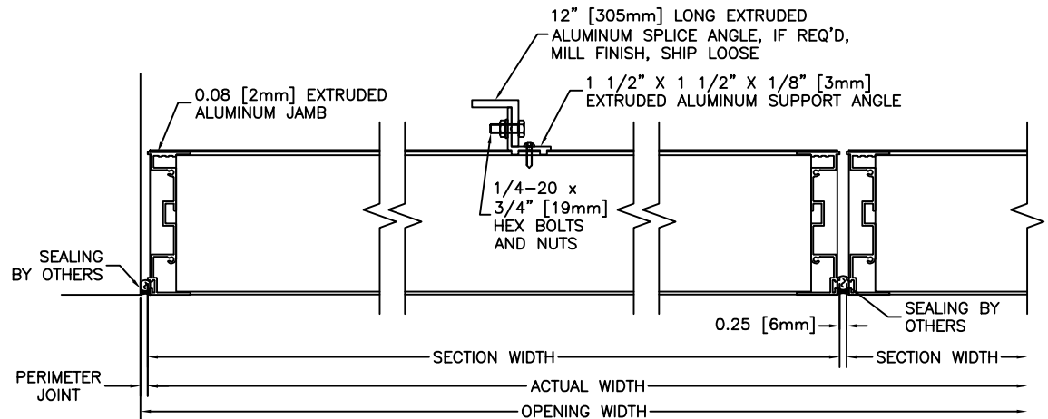
JAMB DETAIL
