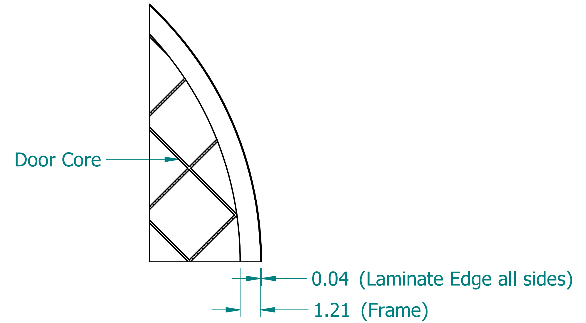
SECTION A-A
