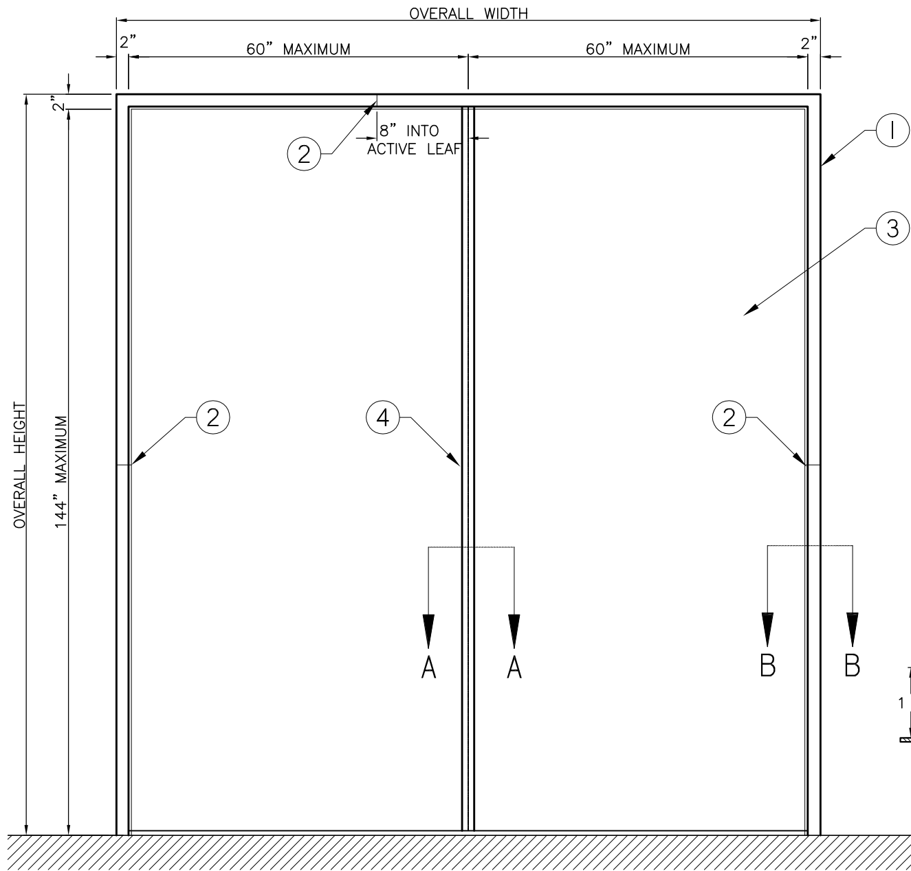
FRAME ELEVATION
