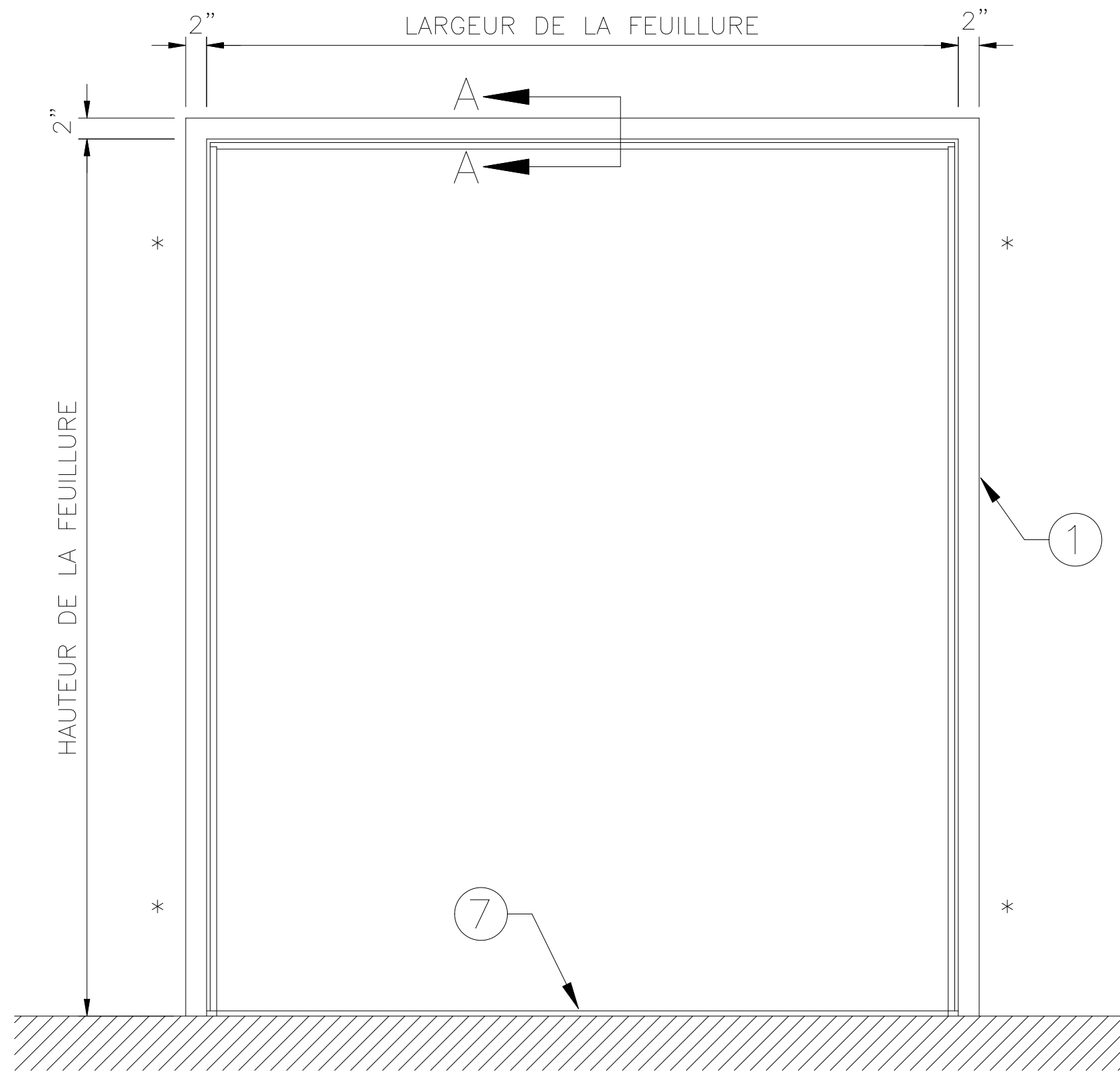
ÉLÉVATION
