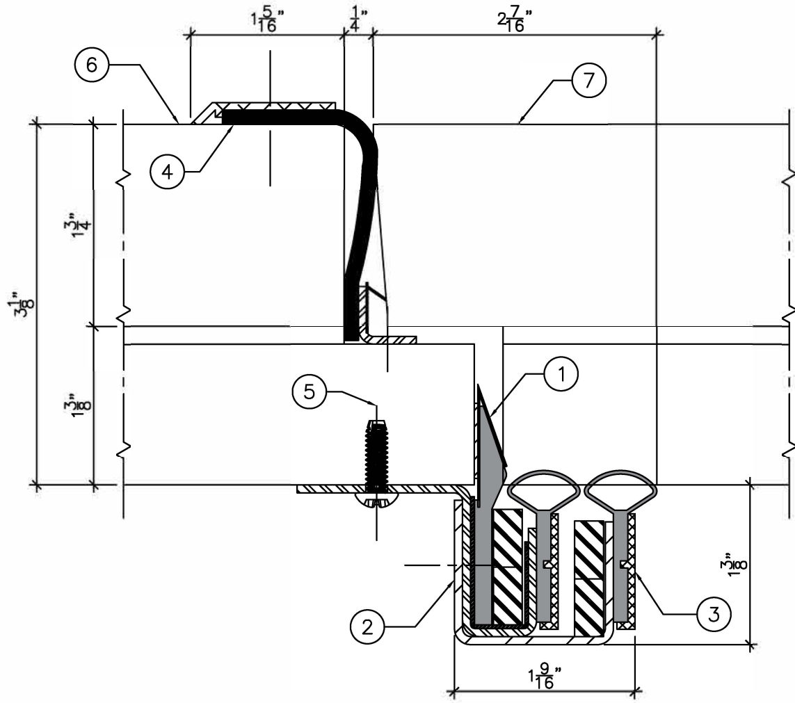
ASTRAGAL SECTION 1'-0" = 1'-0"
