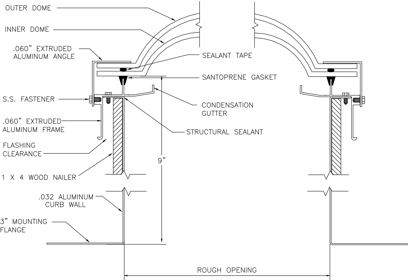
9" EZ SELF FLASHING (MODEL EZSF-9)
