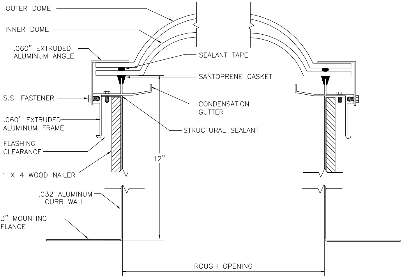
12" EZ SELF FLASHING (MODEL EZSF-12)
