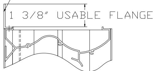
FLANGE FRAME
