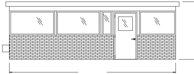
ELEVATION A
