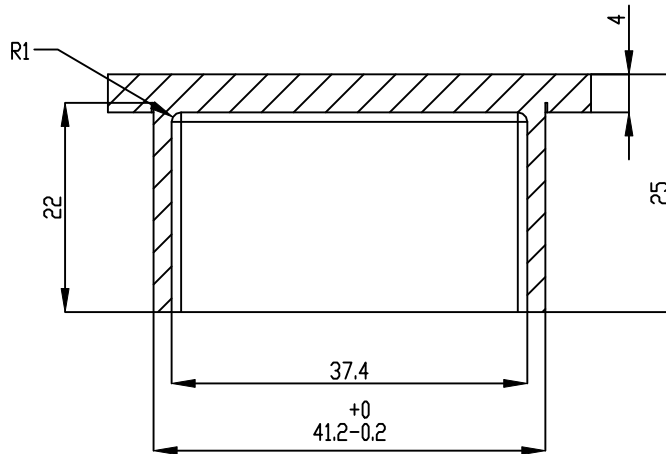
SECTION A-A SCALE 2 : 1.5
