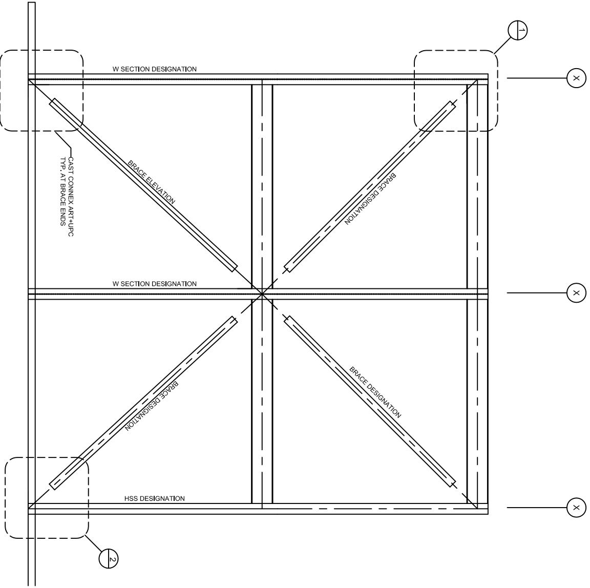
ELEVATION
