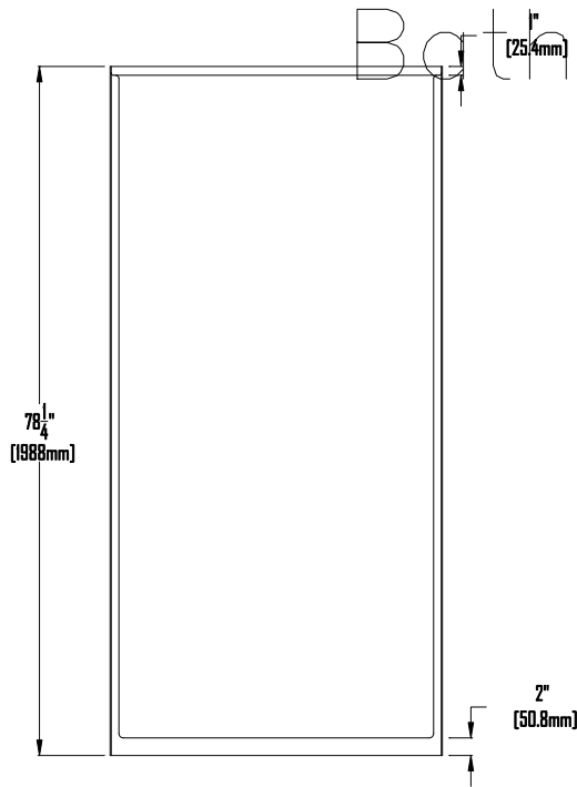
ELEVATION
