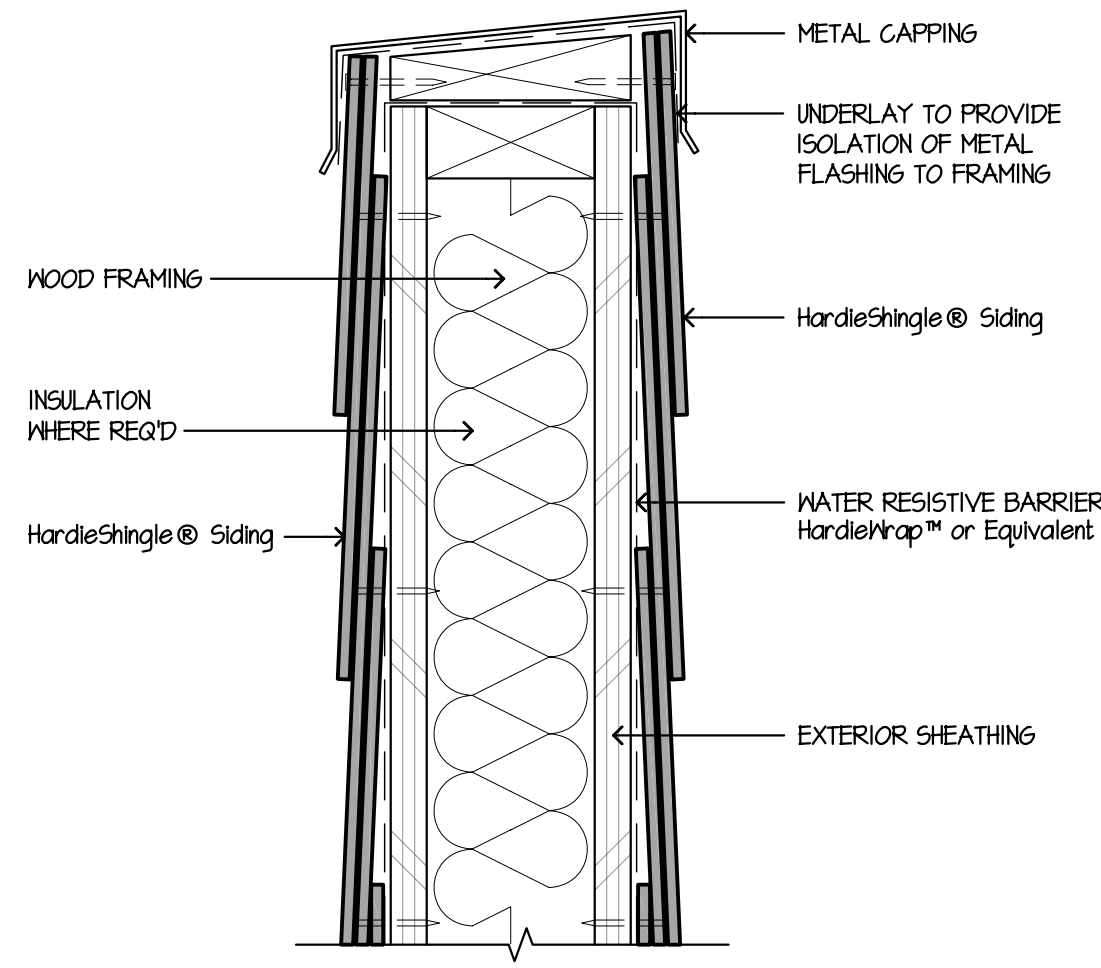
9 PARAPET SCALE: 3/4"=1'-0"
