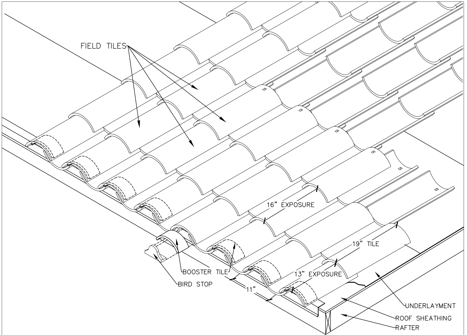
MCA - 8" STRAIGHT BARREL - OVERALL N.T.S.
