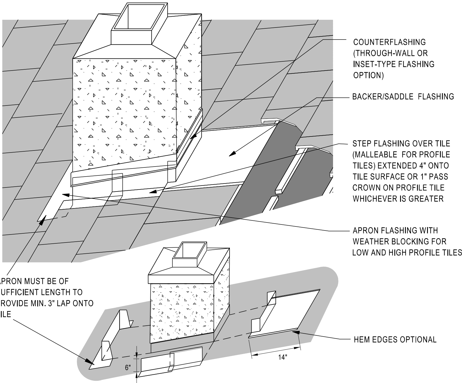
APRON FLASHING
