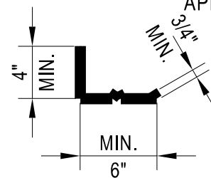
OPTIONAL PAN FLASHING
