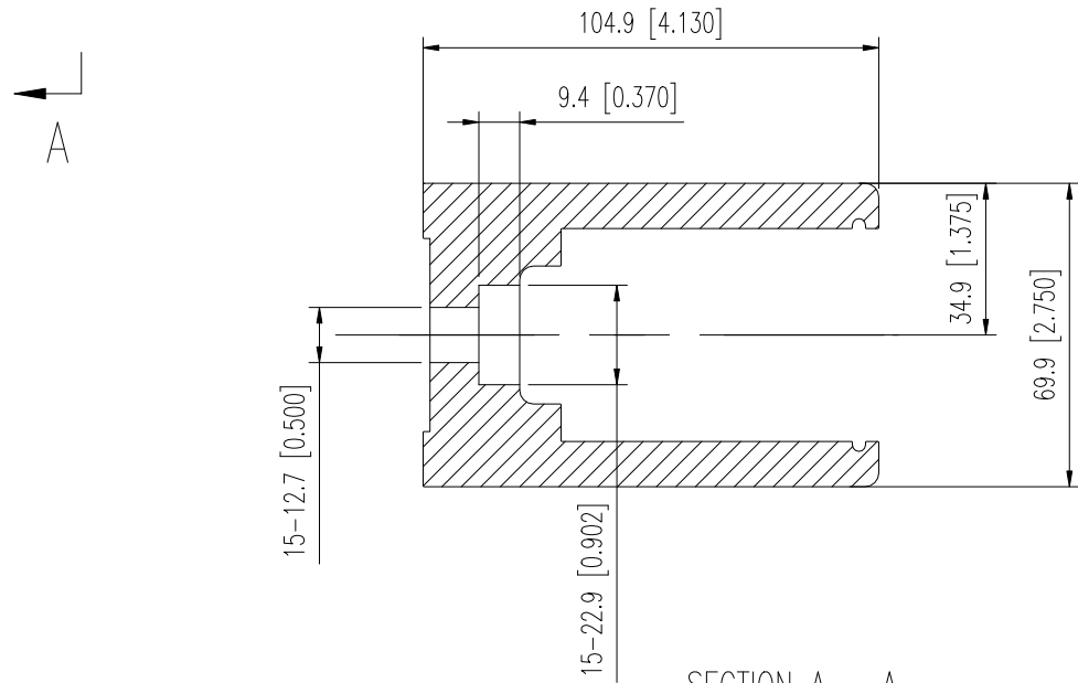
SECTION A - A 1 : 1
