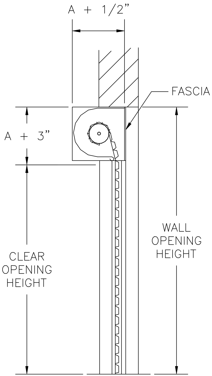
SECTION A-A
