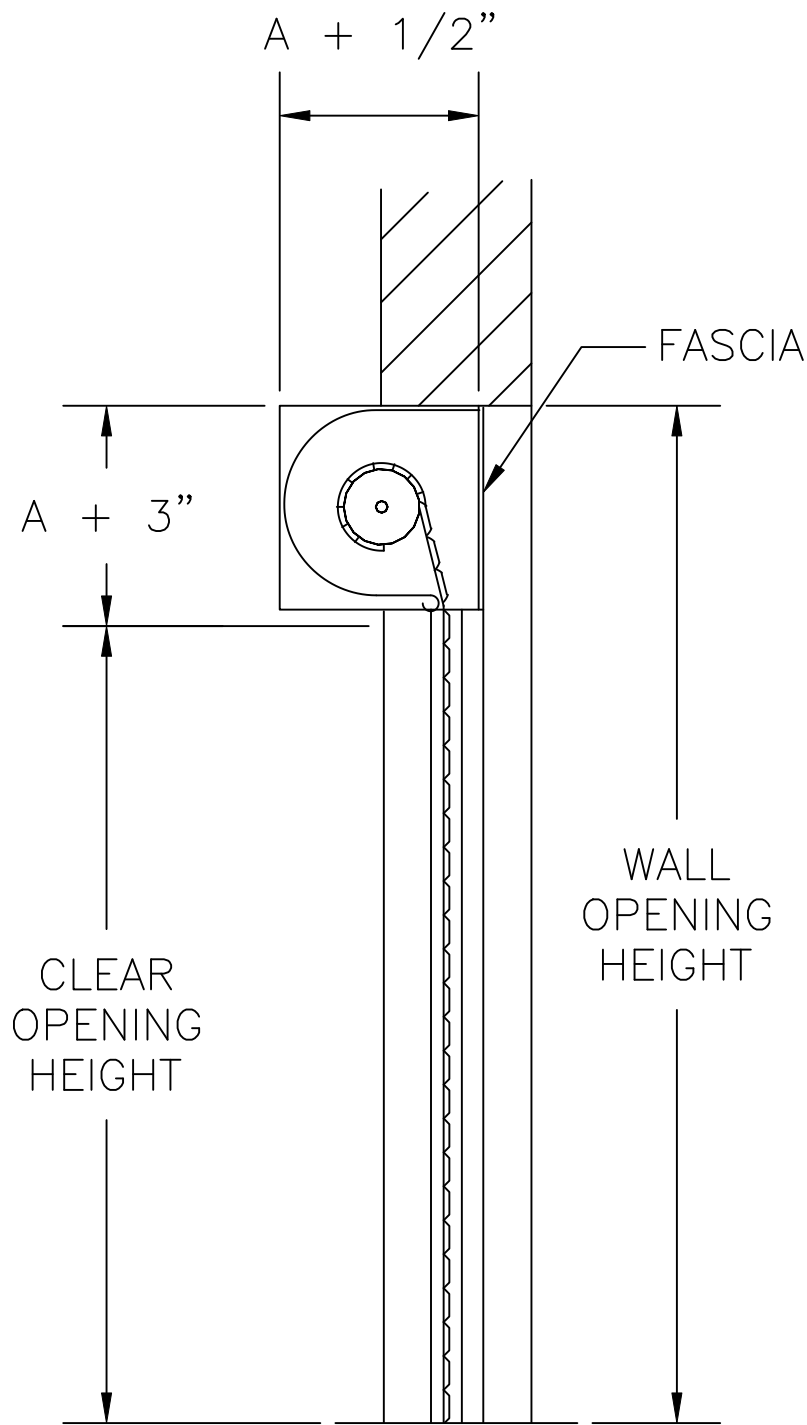
SECTION A-A
