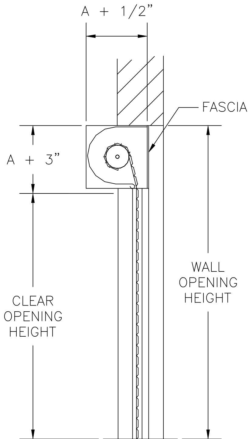
SECTION A-A
