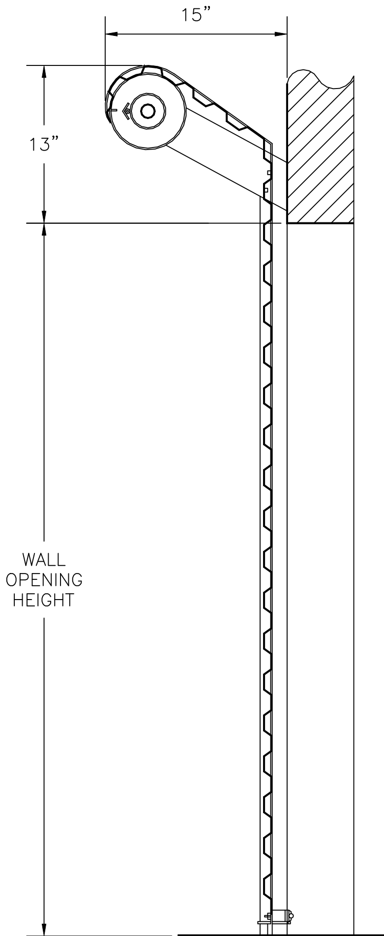
SECTION A-A
