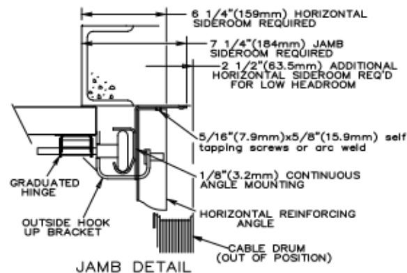
JAMB DETAIL
