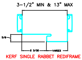
KERF SINGLE RABBET REDIFRAME
