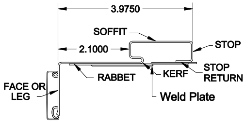
KERF 1-3/4" DOOR BASE
