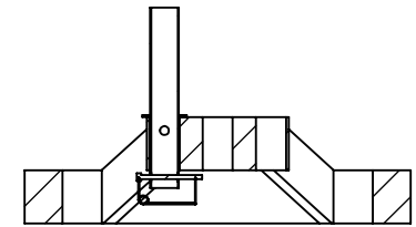
SECTION A-A SCALE 1 : 12
