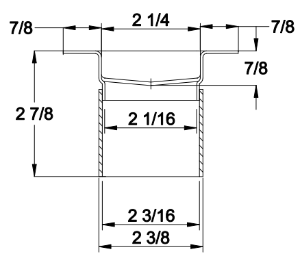
A-A (1:1)
