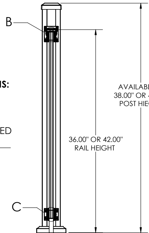
SECTION A-A SCALE 1 : 10
